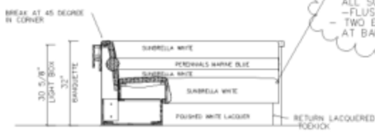
② ELEVATION
