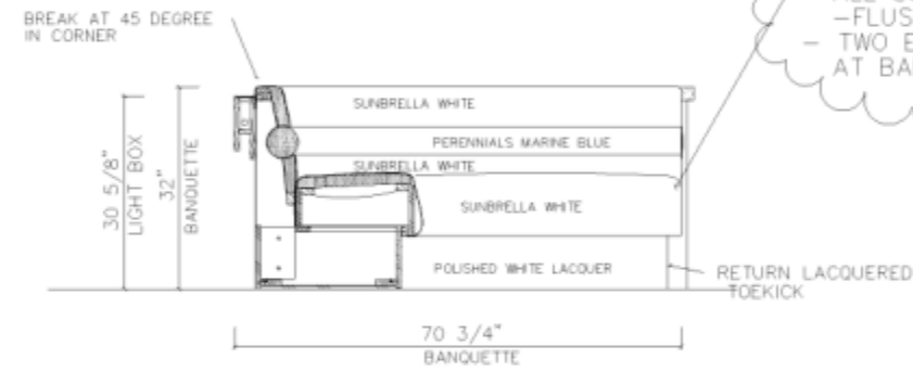
2 ELEVATION SCALE: 3/4" = 1' 0"
