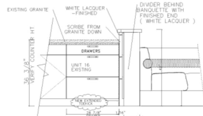
4 ELEVATION SCALE: 3/4" = 1' 0"
